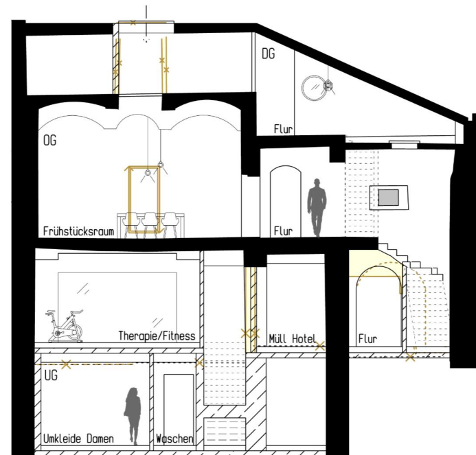
Schnitt © Aris Architekten Anglhuber + Reithmeier PartGmbH
