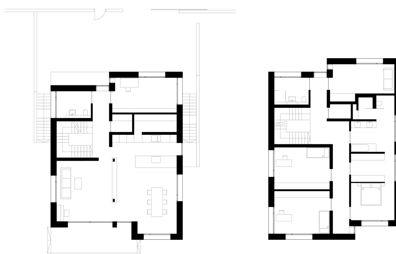
Erdgeschoss und Obergeschoss © SLG Architekten
