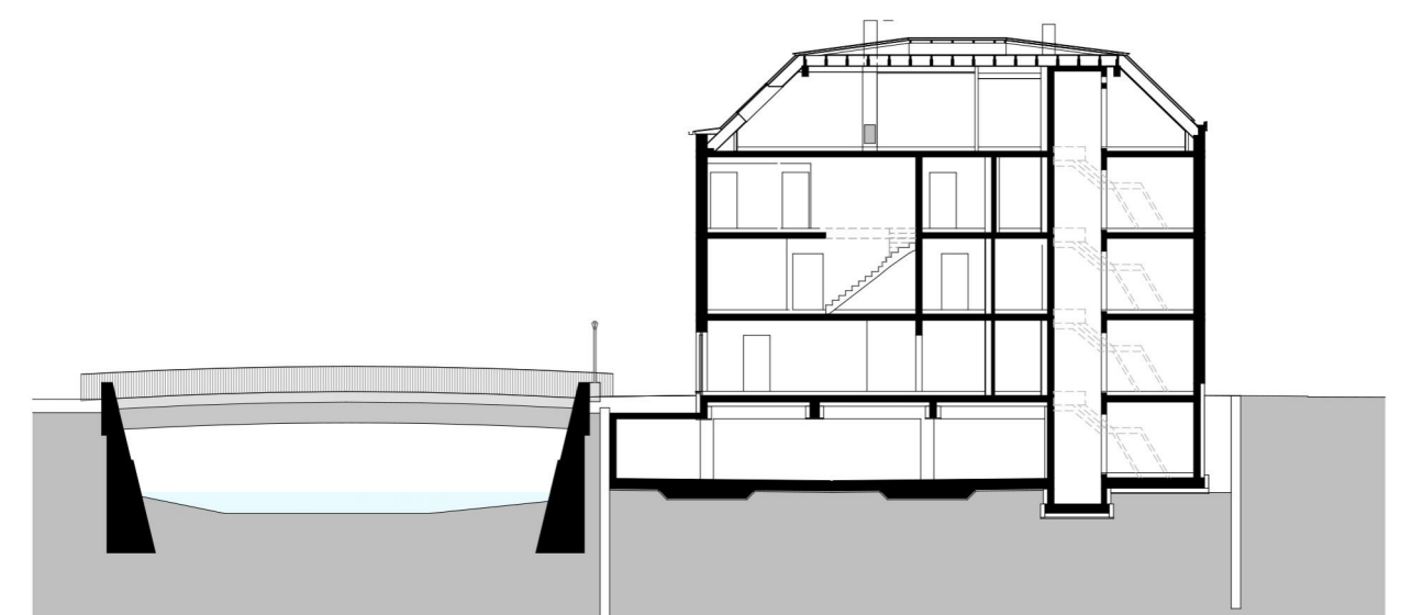
Längsschnitt © F. Krusche
