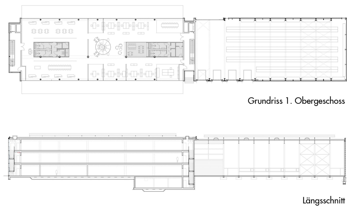
Grundriss und Schnitt © Widmann Architekten
