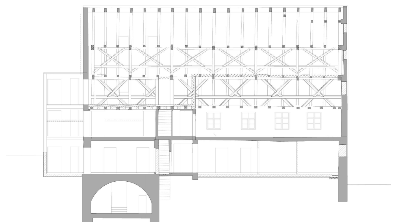
Laengsschnitt © Architekten Claus + Forster PartGmbB
