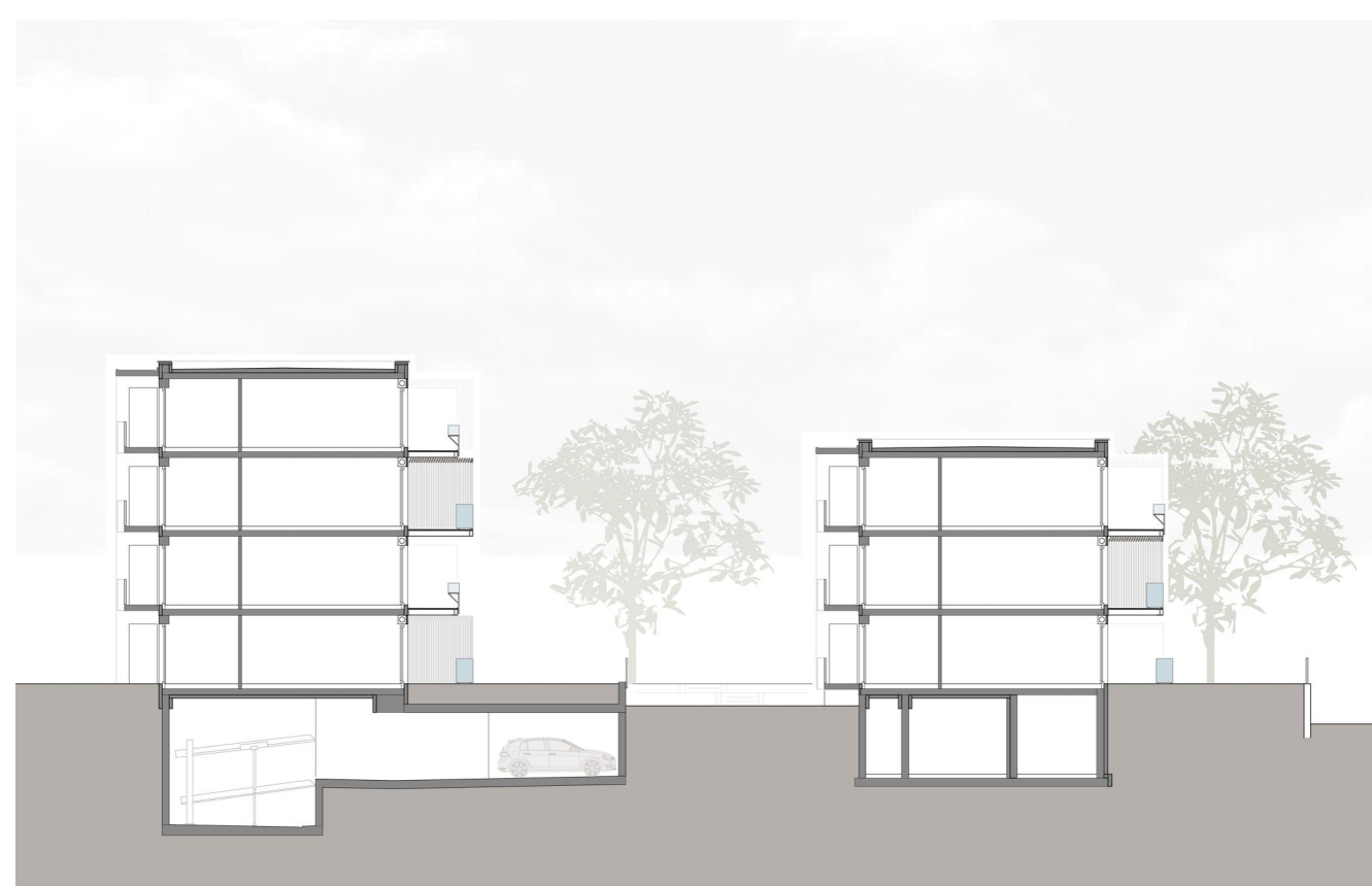
Schnitt © Meyer Huber Architekten Part mbB
