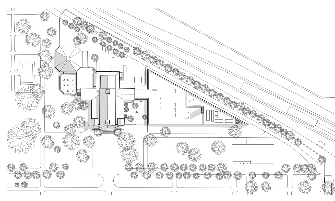
Lageplan © Beer Bembé Dellinger Architekten
